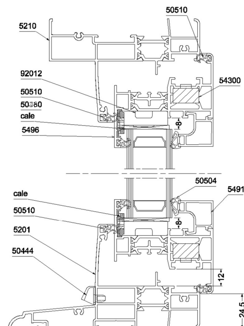
Ouvrant visible Classic+
