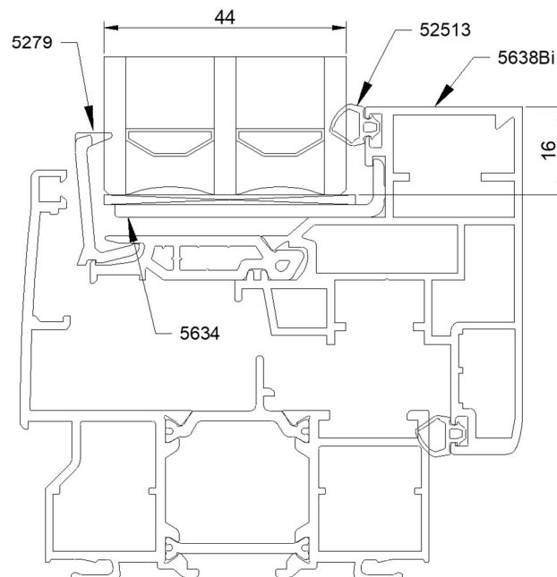
Parclose 5279 - Vitrage 44 mm maximum
