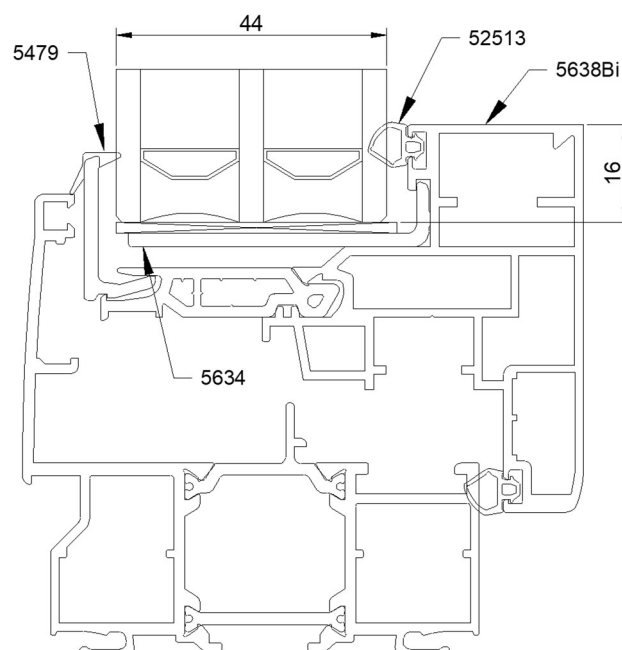
Parclose 5479 - Vitrage 44 mm maximum
