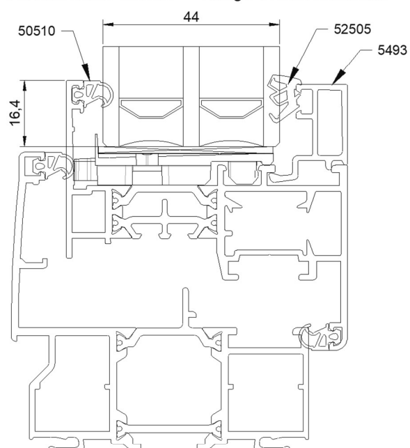
Ouvrant visible Classic+ - Vitrage 44 mm maximum
